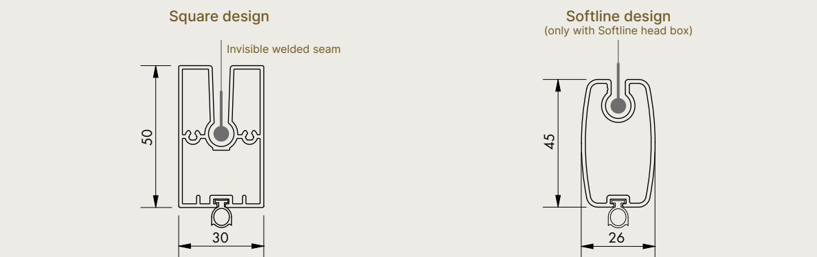
Fixscreen® 100 - Bottom bar
