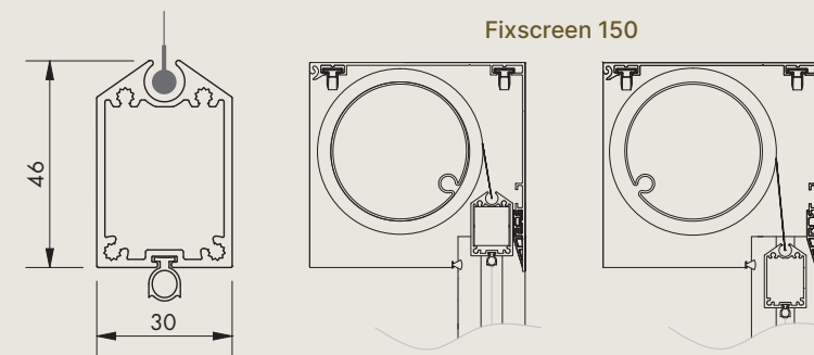
Bottom bar
