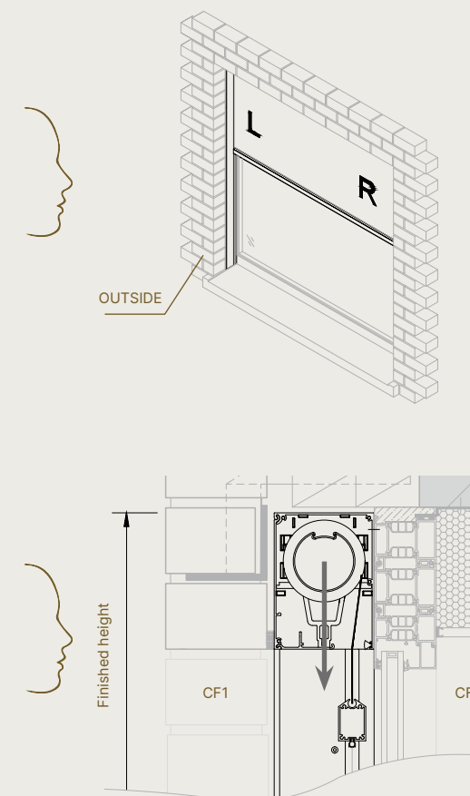
Fixscreen® IM 1 (+) (Solar), IM 7A Fixscreen® Minimal IM 1 (Solar), IM 7A/B, Curtain Wall 50 Panovista® (Max)
