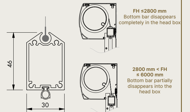
Fixscreen® 150 - Bottom bar
