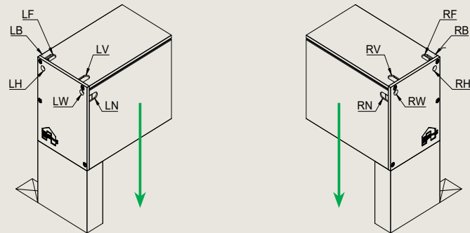
Cable feed - IM 7A
