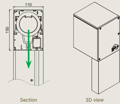
Fixscreen® 100 Slim - IM 7A - Head box
