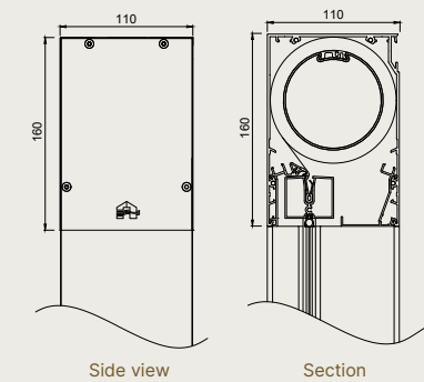
Large - IM 7B - Head box
