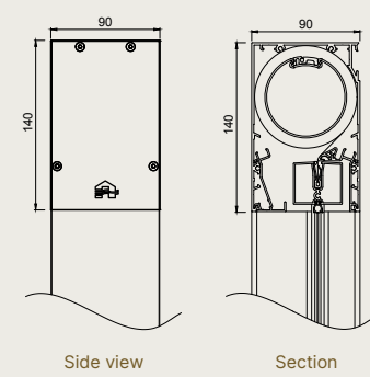
Small - IM 7A - Head box
