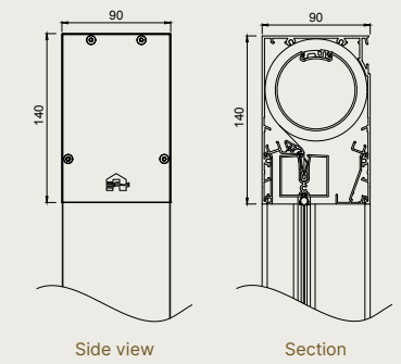
Small - IM 7B - Head box
