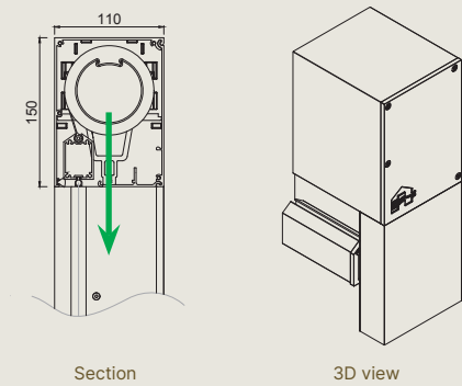
Fixscreen® 100 Slim - IM 7B - Head box
